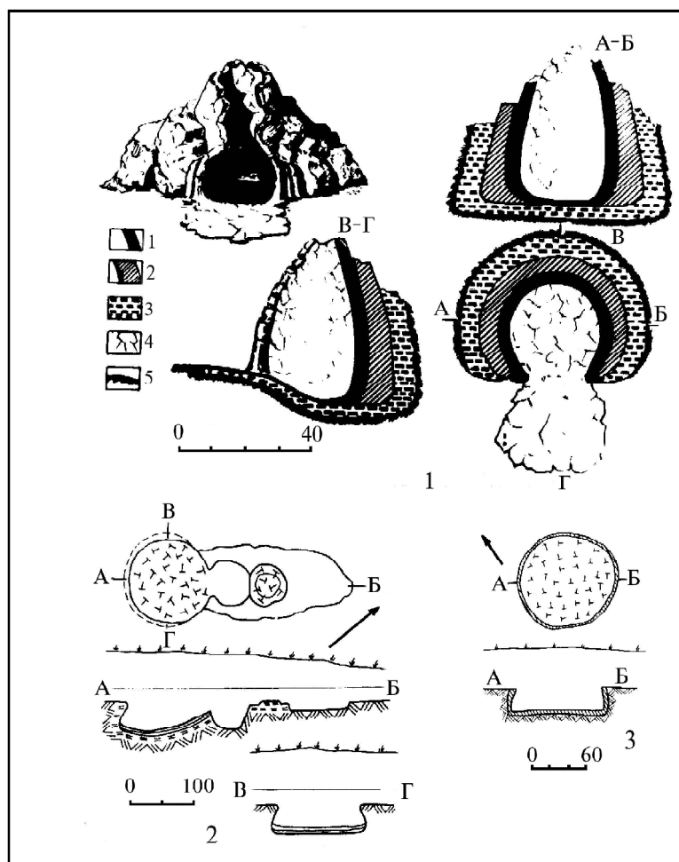
Рис. 5. Железодельательные сооружения поселения Скок: 1 — общий вид, план и разрезы сыродутного горна 2. Условные обозначения: 1 — первый слой обмазки; 2 — второй слой обмазки; 3 — обожженный материк; 4 — обожженная обмазка; 5 — материк. 2. план и разрез печи 1; 3 — план и разрез ямной печи 16.
