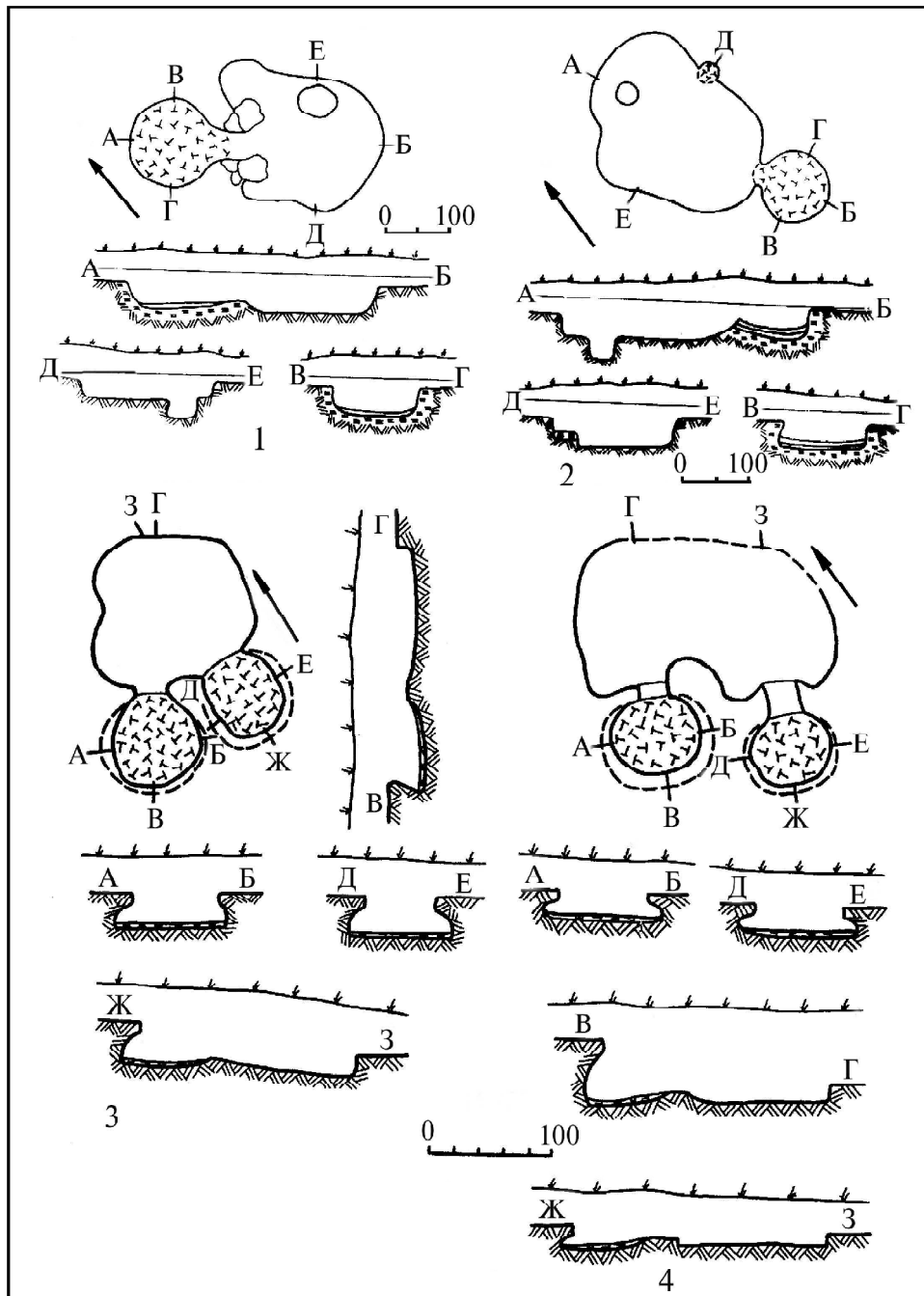
Рис. 4. Планы и разрезы сооружений с купольными печами: 1, 2 — сооружения с одной печью; 3, 4 — сооружения с двумя печами.
