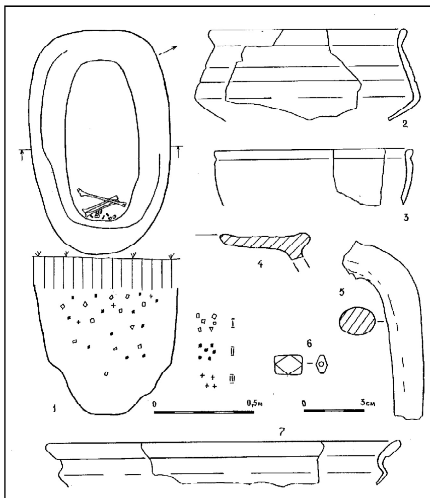
Рис. 3. Погр. 1. 1 — план (I — керамика, II — угольки, III — кальцинированные кости); 2-5,7 — керамическая посуда; 6 — сердоликовая бусина.
