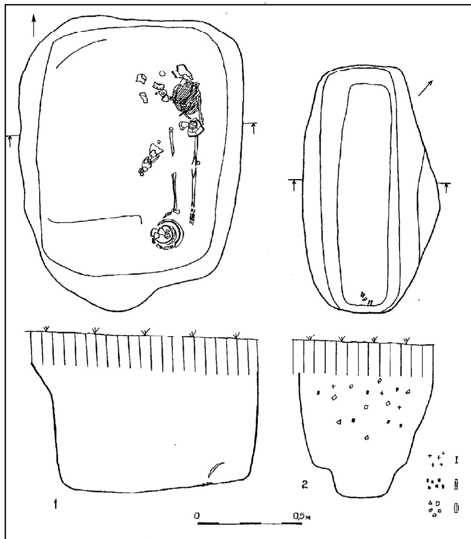
Рис. 4. 1 — план погр. 3; 2 — план погр. 2 (I — кальцинированные кости, II — угольки, III — керамика).
