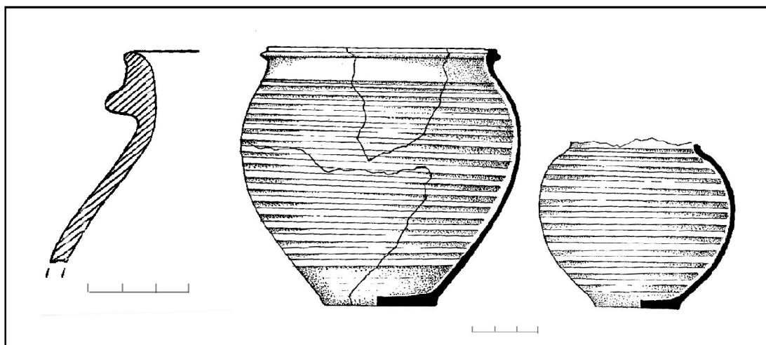
Рис. 4. Гончарные сосуды из конструкции горнов в Лепесовке.
