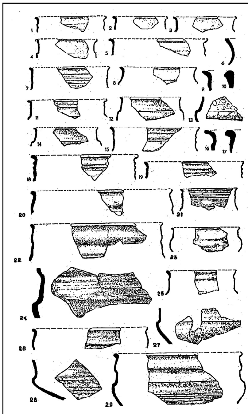
Табл. 18. Керамика поселения Цветау в Саксонии (Meyer 1971).
