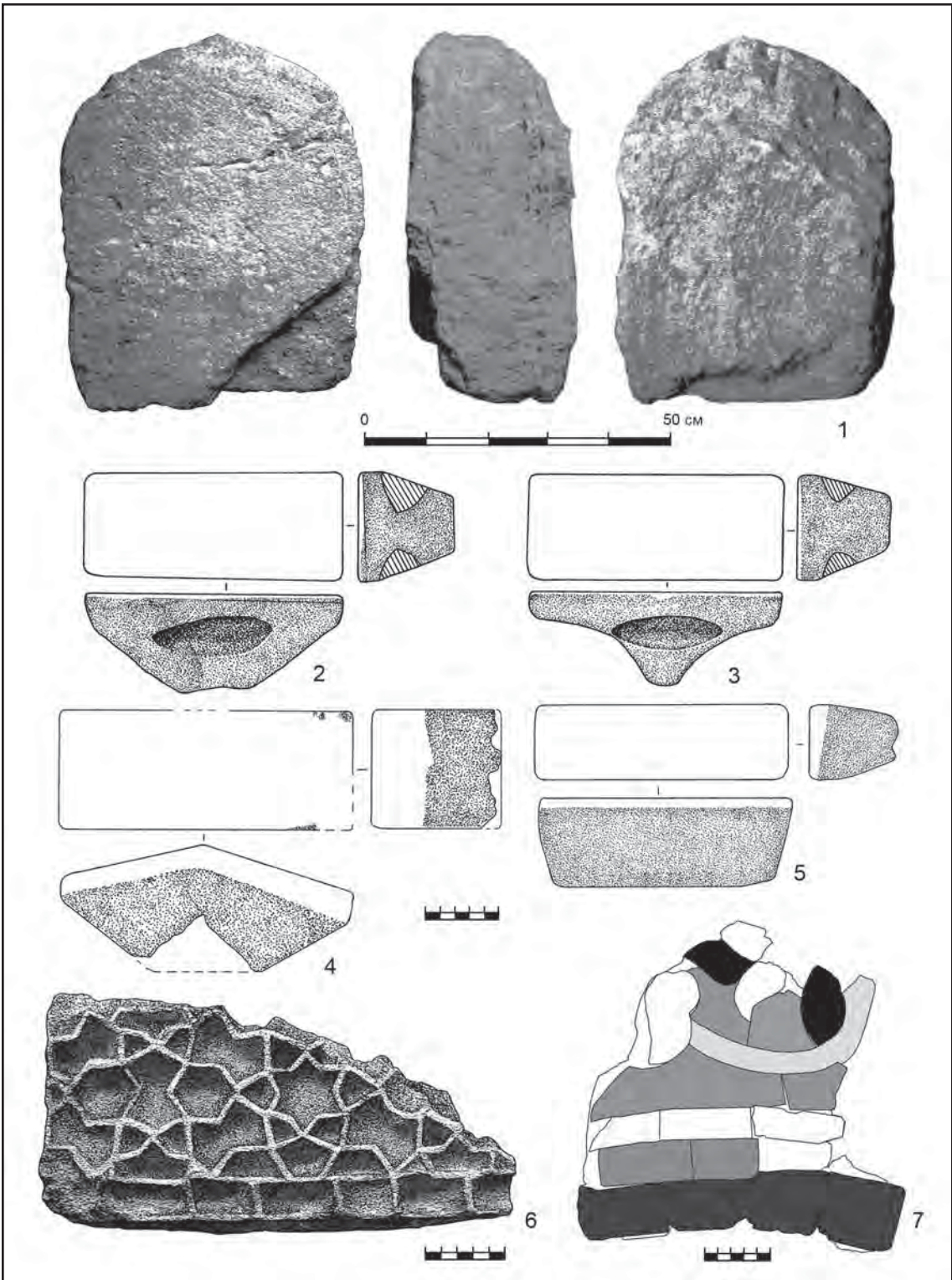
Рис. 18. Городище Конские Воды. Строение 1: 1 — фрагмент надгробия (фото автора); 2—5 — кашинные кирпичи; 6, 7 — типы орнаментов (по Ельников 2017: рис. 2; 3; 4; 1; 10: 1).
