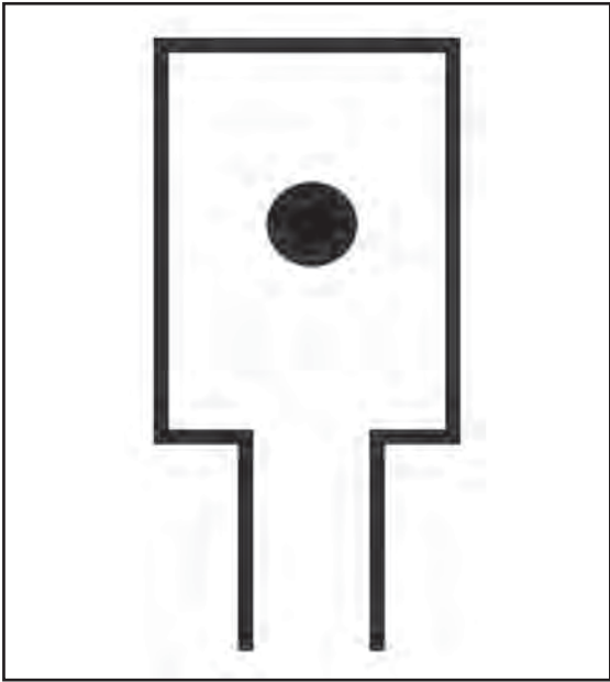
Рис. 3. План печи типа II-a по типологии А. Харизанова.
