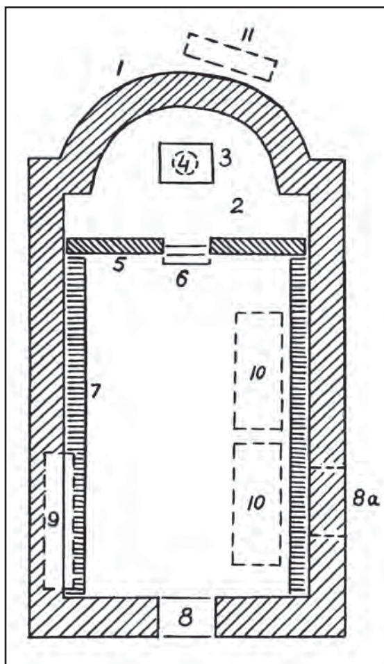
Рис. 4. Обобщенный тип средневекового одноапсидного храма на Южном берегу Крыма: 1 — апсида (обычно полукруглая, редко гранная); 2 — алтарное возвышение (нередко вровень с полом нефа); 3 — престольный камень; 4 — углубление под престолом для мощей; 5 — предалтарная преграда («царские врата», иконостас); 6 — ступени (не всегда); 7 — боковые скамьи — уступ в кладке основания стен (не всегда); 8 — вход (часто сбоку, в положении 8a); 9 — аркосолий в стене (в этой или в противоположной, довольно редко); 10 — могилы в полу (часто в других пунктах, вообще не всегда); 11 — погребения младенцев (или сбоку, вообще не всегда) (по Фирсов 1970: рис. 2).
