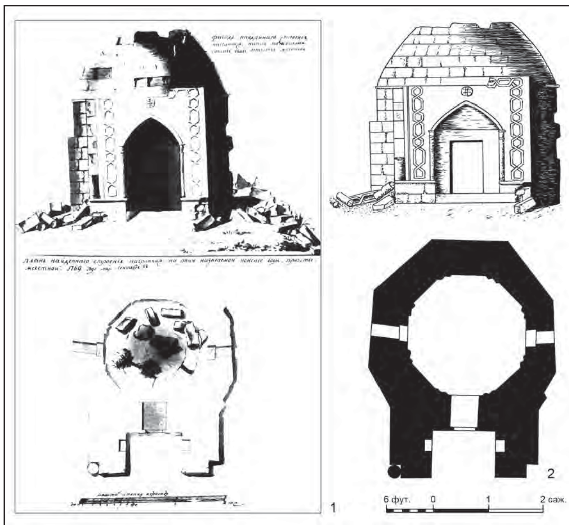
Рис. 8. «План и фасад строения, найденного на берегу реки Конские воды при устье Мечетной. 1769 года, месяца сентября 28»: 1 — РГВИА. Ф. 418. Оп. 1. Д. 1158; 2 — прорисовка автора.
