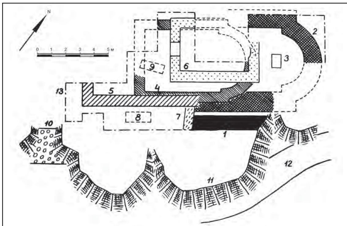
Рис. 10. Серия последовательных по времени средневековых одноапсидных храмов на скале Панея (Паная, Панагия) в Симеизе. Раскоп О.И. Домбровского, 1966 г., документация Л.В. Фирсова, 1966—1967 гг. (один из вариантов интерпретации): 1 — остаток стены, по-видимому, самого раннего храма; 2 — ранний храм с мраморным полом; 3 — престольное углубление раннего храма; 4 — храм с гранной апсидой и мозаичным полом; 5 — поздний храм с мраморным полом; 6 — наиболее поздняя безапсидная капелла или часовня; 7 — поперечная стенка; 8 — могила; 9 — могила другой ориентировки; 10 — остатки боевой стены; 11 — край скального обрыва; 12 — современная дорожка над водосточным каналом (по Фирсов 1970: рис. 6).
