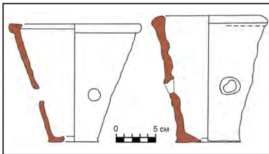
Рис. 10. Сосуды/конусы в древнем садоводстве (по Barat, Morize 1999: Fig. 13: E).
