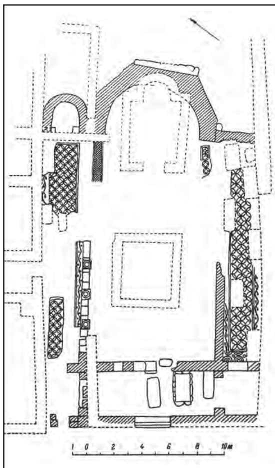
Рис. 11. Херсонесская базилика, раскопанная в 1932 г. Обмер В. Е. Веймарна (по Якобсон 1959: рис. 84).
