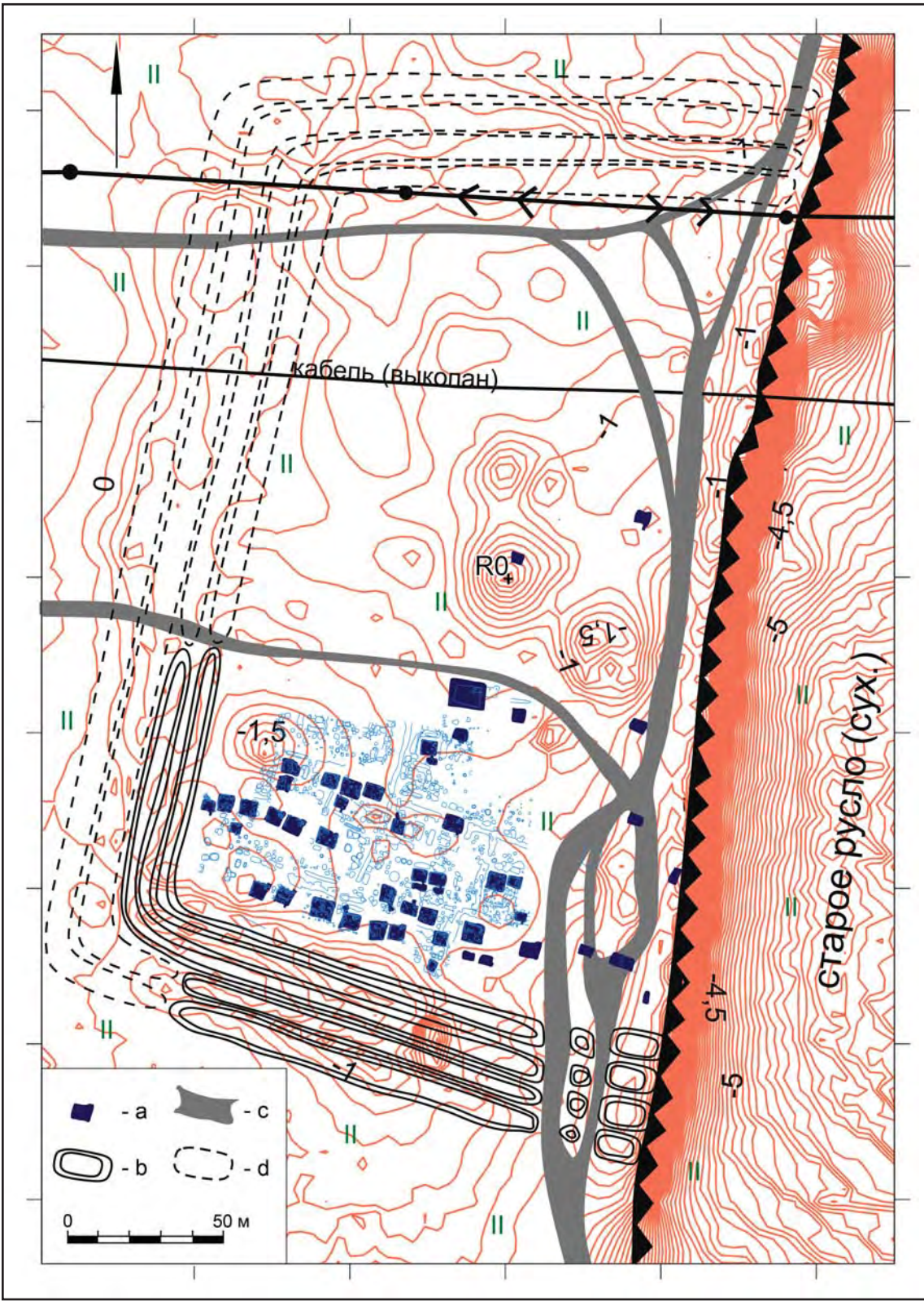
Рис. 1. Иволгинское городище. Условные обозначения: а — жилище; b — вал; c — дорога; d — условно вал. Высоты условные. Сплошные горизонталы проведены через 0,1 м (план выполнил С.Д. Прокопец, 2016).
