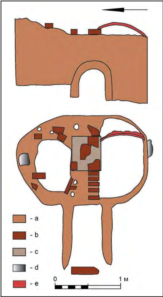
Рис. 2. План печи. Условные обозначения: а — обожженная глина; b — строительная керамика; c — обмазка; d — камни; e — пифос.
