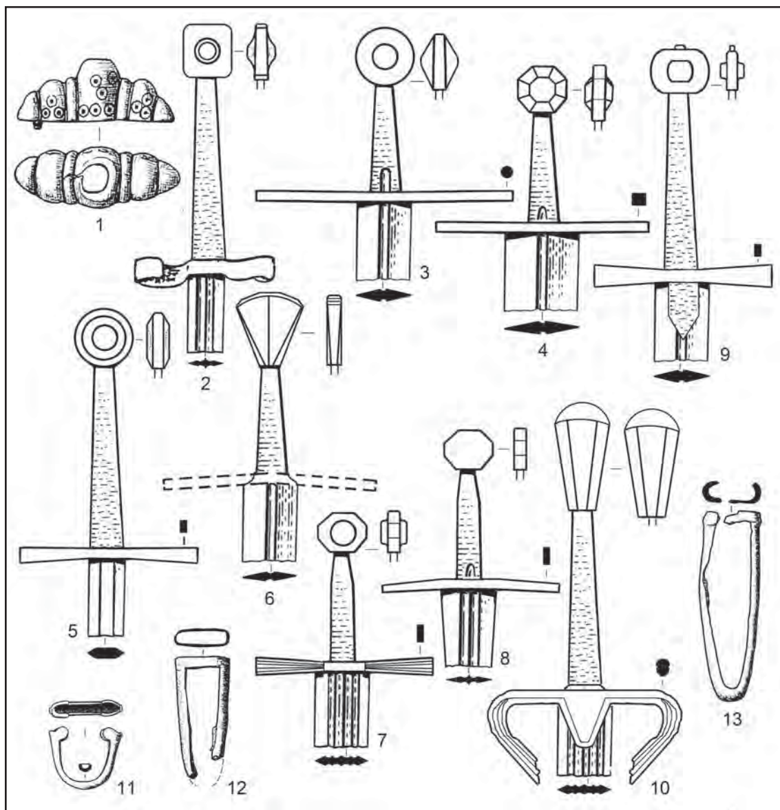
Рис. 2. Прорисовки рукояток, наверший, перекрестьев и наконечников ножен (1, 11—13 — по Пивоваров, Калининченко 2016: 368; 2—10 — прорисовки автора).
