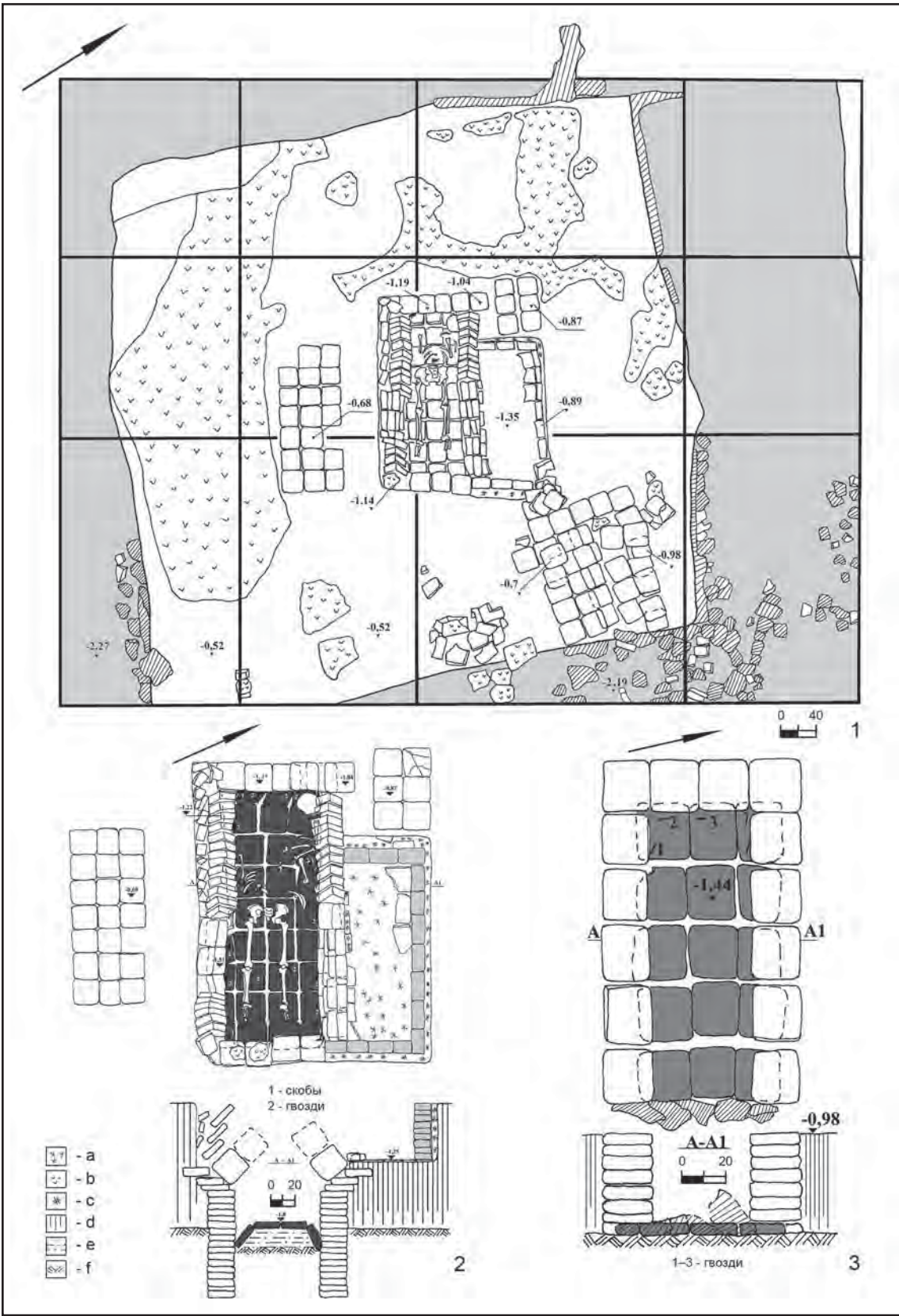
Рис. 17. Городище Конские Воды. Строение 1: 1 — погребальная площадка; 2, 3 — планы погребений; а — песок; b — гипсовая обмазка; с — алебастр; d — чернозем; e — кристаллы мела; f — материк (чертеж автора).
