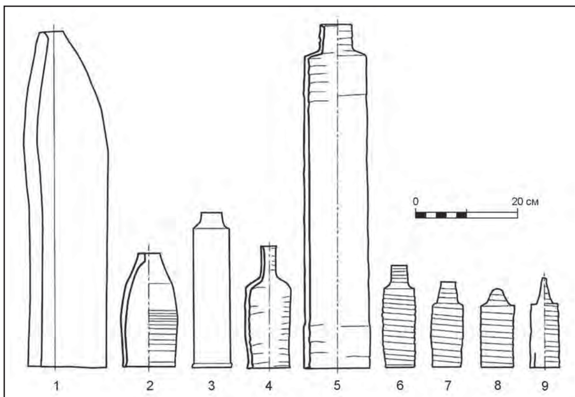
Рис. 13. Схема форм различных труб для конструкции сводов и для купольной конструкции печей (по Lancaster 2012: fig. 9). 1 — Моргантина (Сицилия); 2 — Кабрера-де-Мар (Испания); 3 — Помпеи (Италия); 4 — Утика (Тунис); 5 — Лептис-Магна (Ливия); 6 — Булла-Регия (Тунис); 7 — Карфаген (Тунис); 8 — Фьюмана (Италия); 9 — Римини (Италия).
