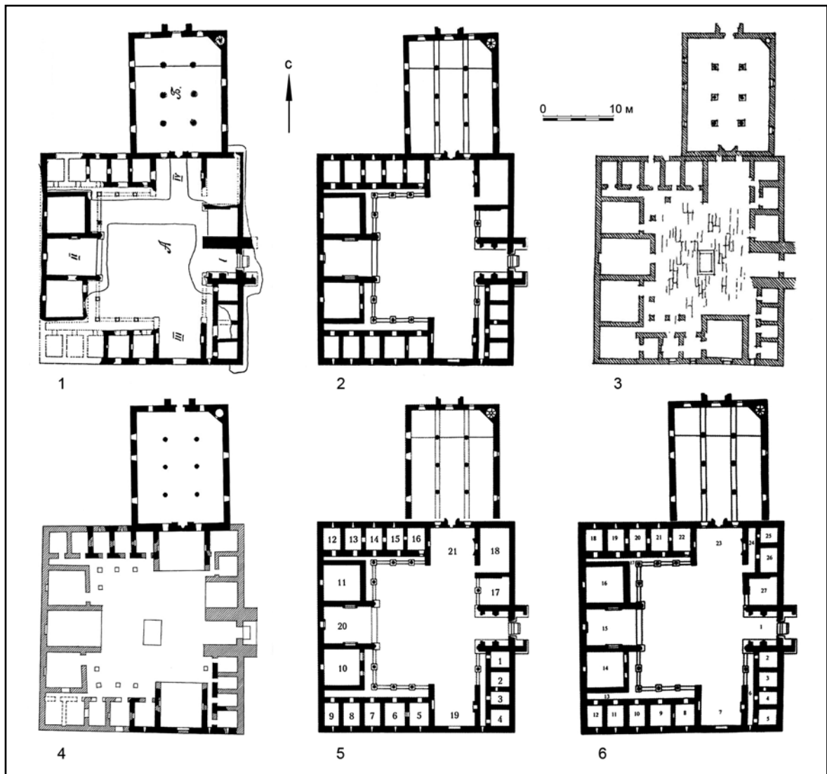
Рис. 1. План солхатского медресе в научных трудах исследователей памятника (1 — по Башкиров 1927: рис. 1; 2 — по Якобсон 1964: рис. 40; 3 — по Крикун 1998: рис. 1; 4 — по Кирилло 2011: рис. 50; 5 — по Крамаровский 2012: рис. 53; 6 — по Зиливинская 2014: рис. 70: 1).
