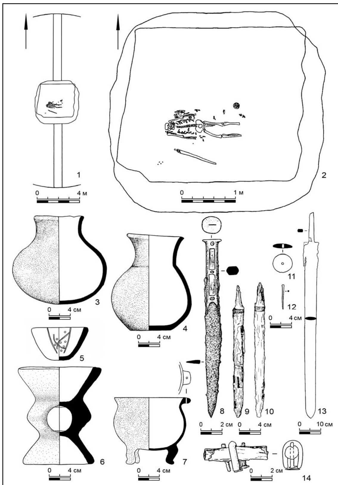
Рис. 2. Погребение кургана №4 могильника Каратобе в Западном Казахстане. 1 — план кургана; 2 — план погребения; 3—6 — керамические сосуды; 7 — медная курительница; 8 — биметаллический нож (бронза, железо); 9, 10 — железные кинжалы; 11 — халцедоновое навершие; 12 — бронзовый штифт; 13 — железный меч; 14 — фрагмент рукояти нагайки.
