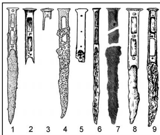
Рис. 3. Биметаллические ножи из Южного Приуралья, Нижнего Поволжья и Средней Азии. 1 — Каратобе; 2 — Агаповский (по Сальников 1950: рис. 34); 3 — Темясковский (по Пшеничнюк, Рязанов 1976: рис. 1: 7); 4 — Целинный I (по Боталов, Гуцалов 2000: рис. 33: 18); 5 — Нижнее Поволжье (по Рау 1927: рис. 25); 6 — Старица (по Шилов 1968); 7 — Бельбек III (по Гущина 1970: рис. 16: 4); 8 — Ворухское ущелье (по Литвинский 1978, рис. 4: 1); 9 — Урюкзор (по Горбунова 1983: рис. 5: 14).
