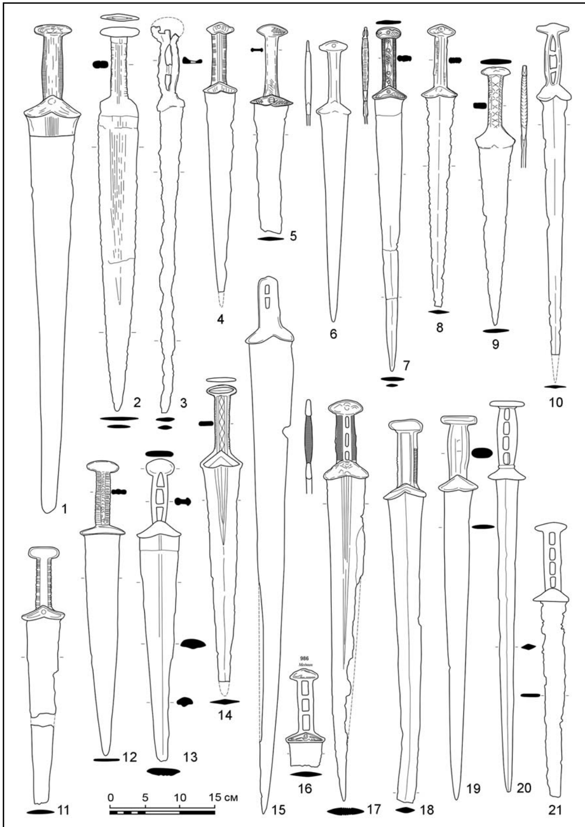
Рис. 3. Акинаки типа Чертомлык: 1 — Житков-II, к. 3, п. 2 (пос. Веселый); 2 — Rogozцы; 3 — Ближнее Стояново, к. 8, п. 1; 4 — Конь-Колодезь; 5 — Сухоносовка; 6 — Чичерино; 7 — Ключ; 8 — Липецкий район; 9 — Красный Лиман; 10 — Сухин; 11 — ГКИМ (дар Терещенко); 12 — Перещегино, к. 12, п. 1; 13 — Бердянский курган; 14 — Кистендей; 15 — Новоселка; 16 — Медвин; 17 — Екатериновка; 18 — Измаил, курган; 19 — Черкасская волость; 20 — Старый Мерчик, к. 3, п. 1; 21 — Ковали; 22 — Львовский музей (рисунки автора по: Апальков 1995: рис. 1: 1; Бандуровский, Буйнов 2000: 77, рис. 8: 7, 8; Березуцкий 1996: рис. 6: 2; Бессонова 1994, рис. 5: 20; Галанина 1977: 53, табл. 33: 3; Клоков 1996: 130, рис. 5: 10; Ковпаненко, Левченко 1977: 60; Косиков, Павлик 1992, рис. 1: 3; Кулатова 1995: 174, 175; Махортых 2012: рис. 13: 1; Медведев 1999,
