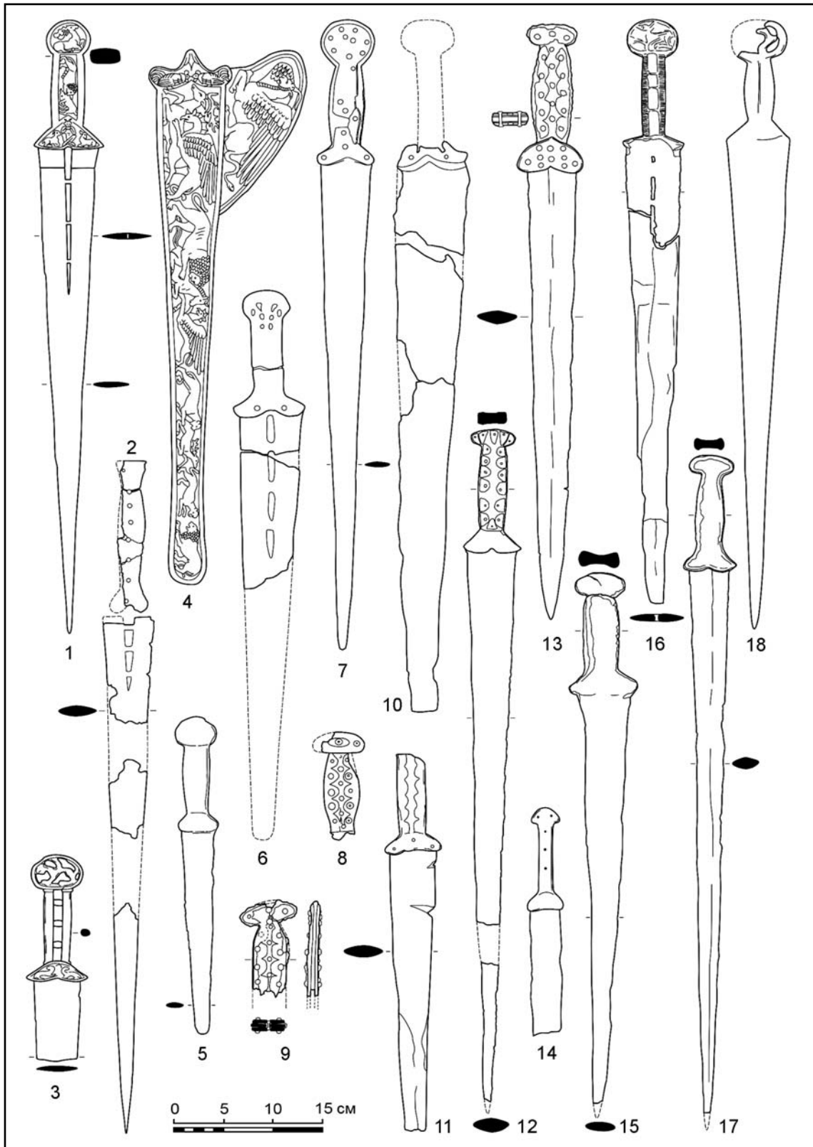
Рис. 2. Акинаки типа Чертомлык: 1, 4 — Толстая Могила; 2 — Капуловка-I, к. 2; 3 — Хвощевая лесная дача (с. Милорадово); 5 — Плискачевка; 6, 10 — Солоха; 7 — Макеевка, к. 489; 8 — Шульговка, I-й курган, меч № 2; 9 — Дудчаны, к. 3, п. 3; 11 — Новорайск; 12, 17 — Дуровка, к. 9; 13 — Белозерка (с. Ильинка), к. 4, п. 2; 14 — Широкое-II, к. 62, п. 1; 15 — Дуровка, к. 10; 16 — Горняцкий; 18 — недокументированный меч из собрания Государственного Эрмитажа; 19 — Каневский уезд (рисунки автора по: Алексеев 2006: рис. 1: 2; Галанина 1977: табл. 10: 21; История Луганского края 2003: 83, рис. 17; Манцевич 1987: 46, кат. 30, 50; Мозолевський 1979: 69—73, рис. 52—56; Петренко 1967: 42, табл. 33: 4, 8; Плешивенко 1991: 61, рис. 6: 3; Пузикова 1969: рис. 6: 3, 4, 5; 2001: рис. 30: 2, 3; Рудинський 1928: 50, табл. VII: 2; Сокольский 1954: 133, табл. II: 2; Тереножкин и др. 1973:
