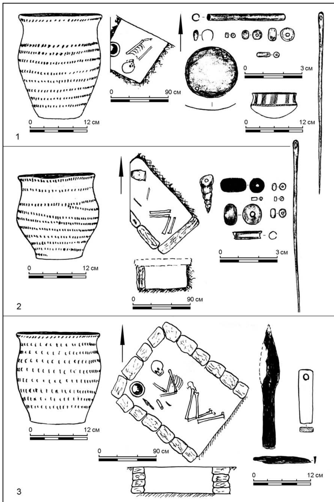
Рис. 8. Горшки, тип 1, вариант 3: могильник Кисловодской мебельной фабрики 1, 1 — п. 30; 2 — п. 32; 3 — п. 19 (по Рунич 1970: рис. 6: 1—6; 1971: рис. 7: 18—28).
