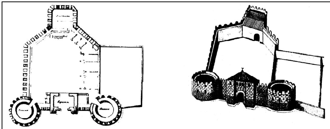
Рис. 2. Чертеж и рисунок крепости, составленные в 1789 г. инженером Фрейганом.
