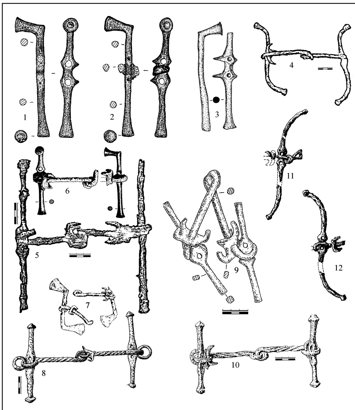
Рис. 3. Детали снаряжения коня. 1—3 — бронза; 6 — железо и бронза; 4, 5, 7—12 — железо. 1, 2 — Журовка, курган 400; 3 — Каменная Балка 6/2; 4 — Стеблев, курган 1; 5 — Стеблев, курган 3; 6 — I Завадская Могила; 7 — Брут, курган 1; 8 — курган 11 группы Частых; 9 — Перещепино, курган 12; 10 — Дуровка, курган 9; 11, 12 — Страшная Могила. 3 — по Ю.С. Гребенникову; 4, 5 — по С.А. Скорому; 6 — по Б.Н. Мозолевскому; 7 — по Т.А. Габуеву, В.Р. Эрлиху; 8, 10 — по А.И. Пузиковой; 9 — по В.Ю. Мурзину, Р. Ролле, В. Херцу и др.; 11, 12 — по В.А. Ильинской.
