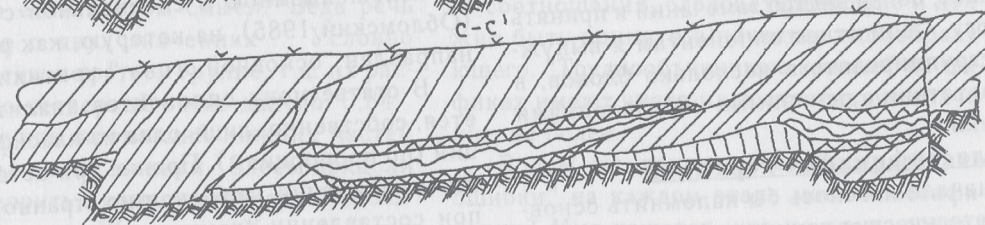
Рис. 14. План замыва и разрезы постр. 10.
